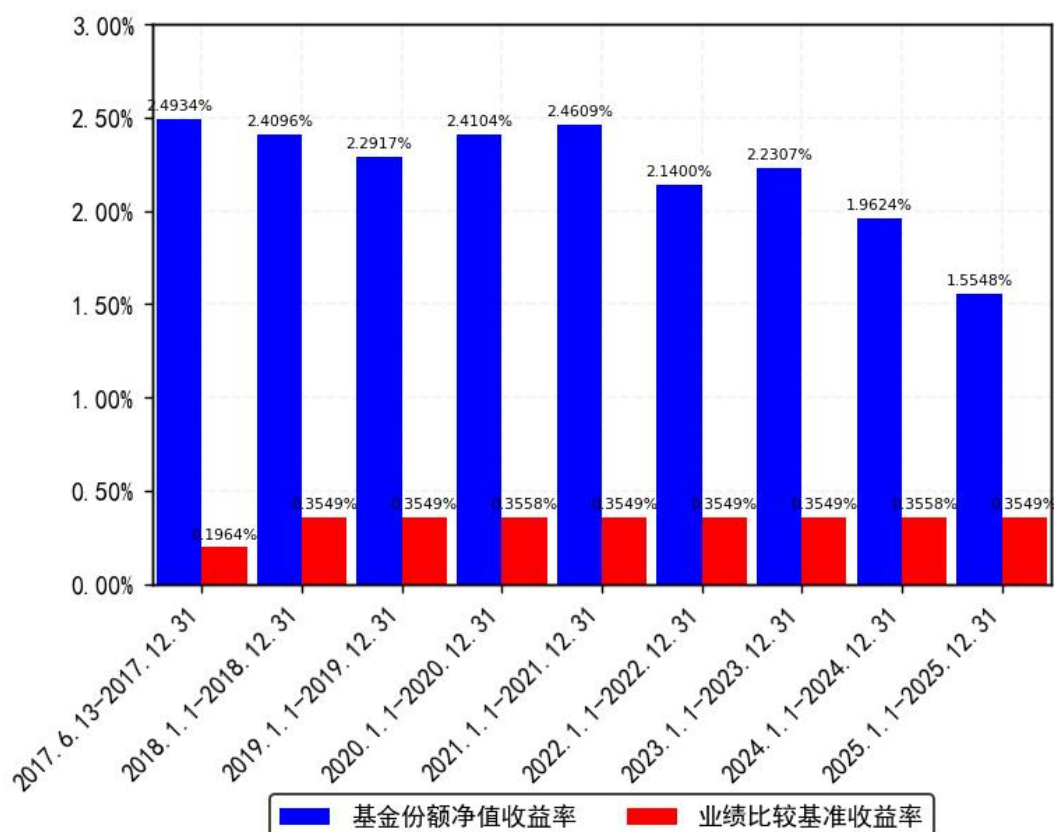
招商招福宝货币B每年净值收益率与同期业绩比较基准收益率的对比图
