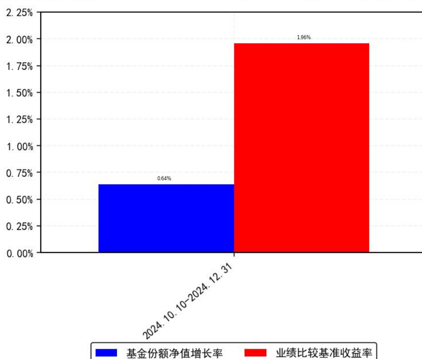
招商智星稳健配置混合（FOF-LOF）D 每年净值增长率与同期业绩比较基准收益率的对比图
